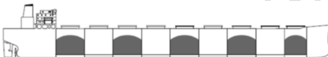
隔舱装载（满载）（摘自《IACS 文件 Rec46rev1》）
